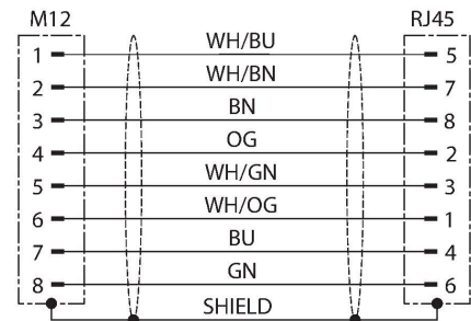
diagrama de conexiones
